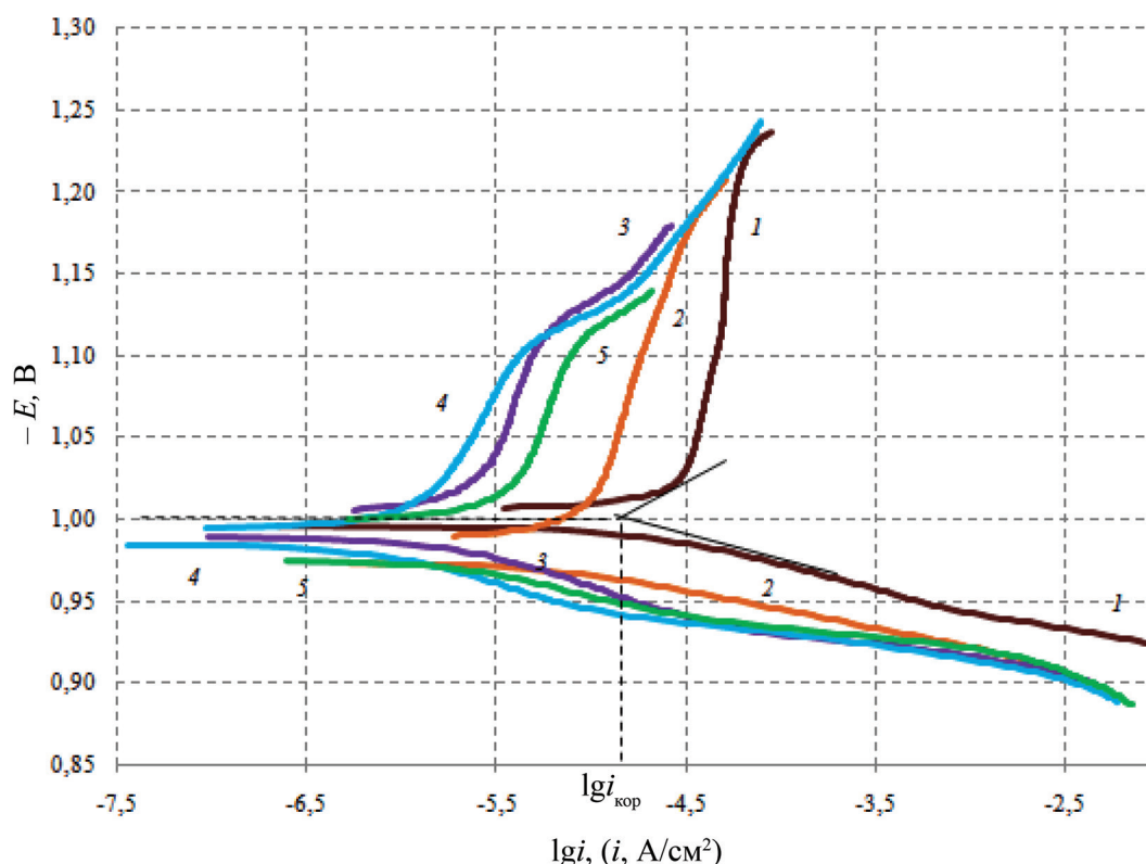
Рис. 3. Поляризационные кривые в 3%-ном растворе NaCl без (1) и с ингибитором \text{Na}_3\text{VO}_4 (2–5) в различных концентрациях: 2 – 0,00005 М; 3 – 0,0001 М; 4 – 0,0002 М; 5 – 0,0003 М
