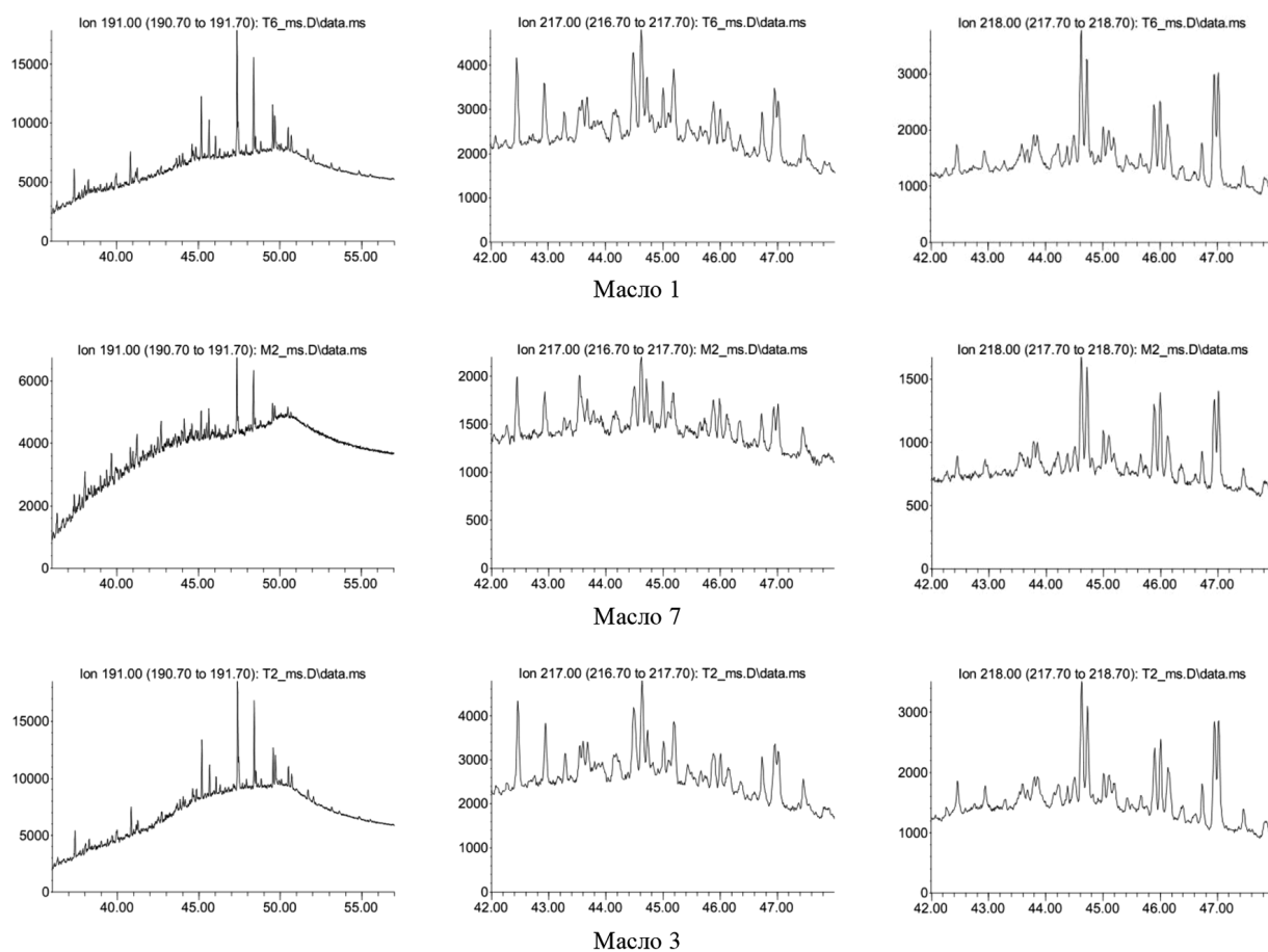
Рис. 6. m/z 191, 217, 218-фрагментограммы (слева направо) моторных масел SAE 10w-40
