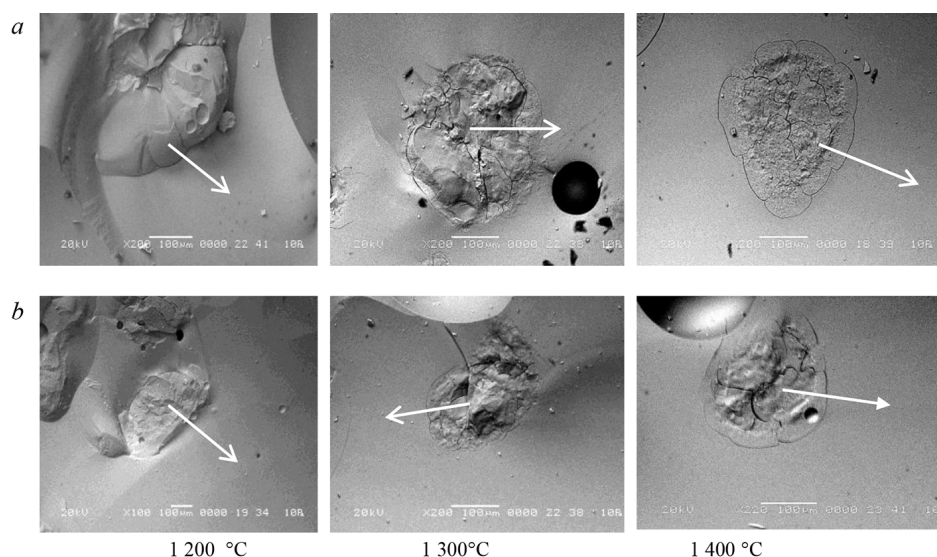
Рис. 3. ЭМ-исследование образцов, синтезированных с использованием кварцевого песка фракции 0,315–0,8 мм при температурах 1 200, 1 300 и 1 400 °C без выдержки (а) и с выдержкой 1 ч (б)
