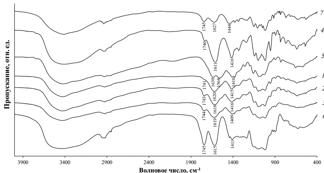
Рис. 5. ИК-спектры пористых материалов на основе ИПЭК Хит-Ag / Пект-Ag 0 (1), Хит-Ag / Пект 0 (2), Хит-Ag / Пект-Ox 0 (3) и их компонентов (Хит-Ag (5), Пект-Ag (4), Пект-Ox (6), Пект (7))
