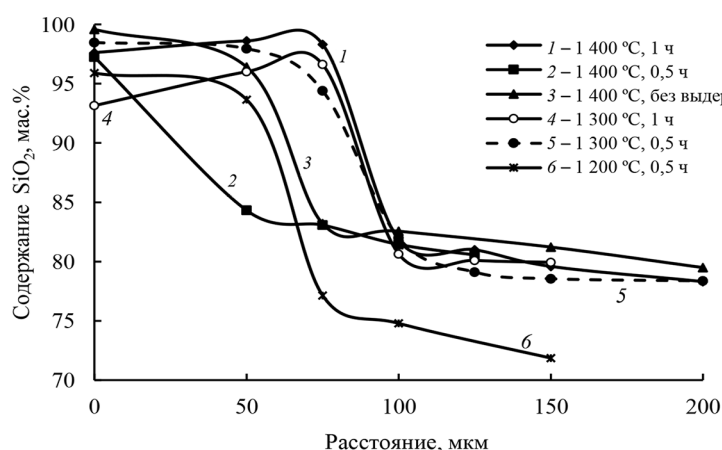
Рис. 4. Изменение содержания \text{SiO}_2 по линии анализа для кварцевого песка фракции 0,315–0,8 мм
